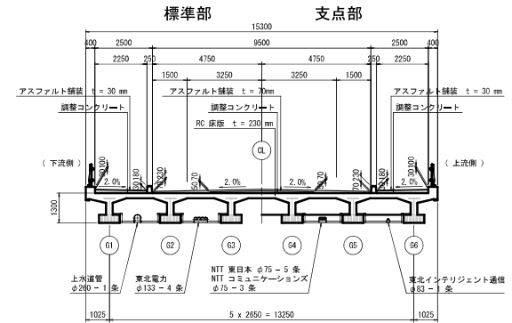
上部工断面图 S=1:100
